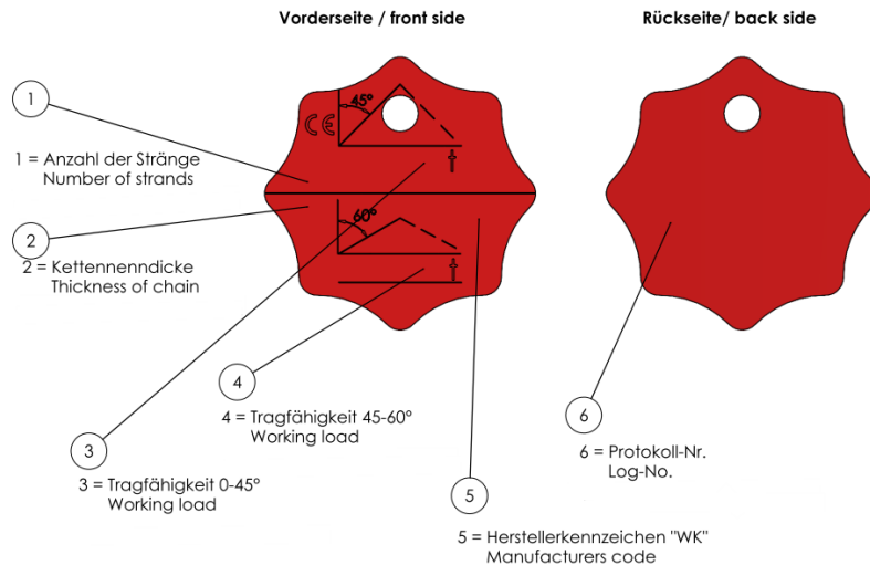
Abb. 2: Mehrstrang Kettenanhänger/ identification tag for multi leg chain gears
